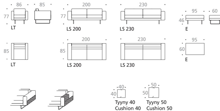
Taivutevaihtoehdot Wooden part alternatives
